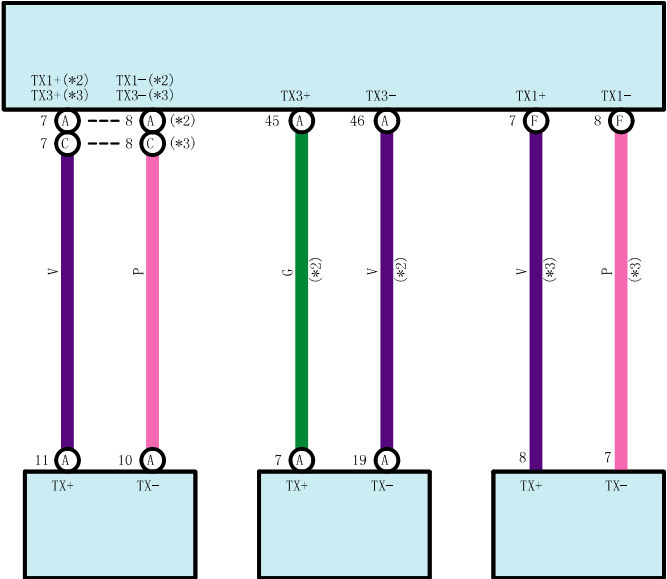
F75 (A) 驻车辅助 ECU
